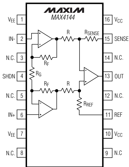
QSOP
