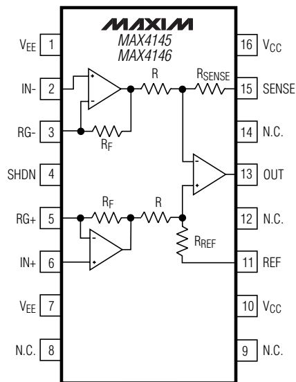
QSOP
